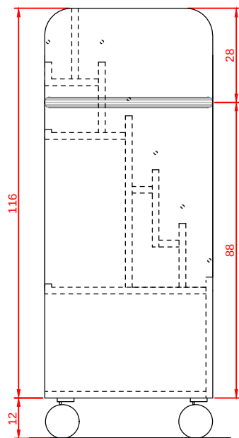
VISTA LATERAL
